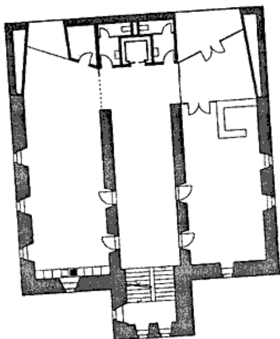
Stockalperturm – půdorys budovy v přízemí (internet: Wiederaufbau Gondo: Durrer Linggi Schmid)
