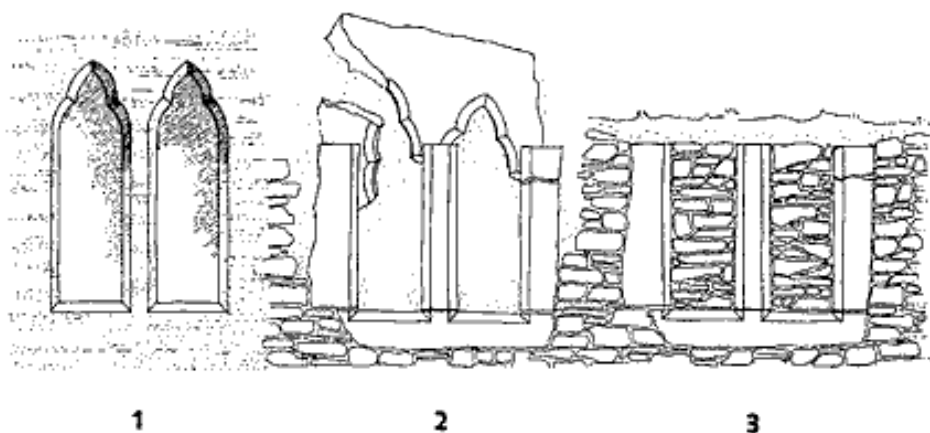
1 2 3 Hrad Šaumburk, raně gotické okno v přízemí dvorního průčelí hradního paláce: 1 – rekonstrukce původního stavu, 2 – stav okna v době provedení archeologického výzkumu v 80. letech 20. stol. (kromě překladu jsou všechny prvky na původním místě), 3 – současný stav po provedení sanace – osazena kopie středního sloupku, provedena konzervace a nutné doplnění hmoty původního zdiva a zřízení ochranné zazdívký (kresba autor 2007)
