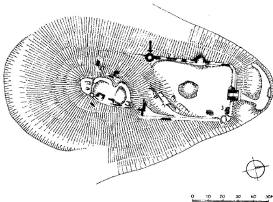
Hrad Křídlo, aktuální půdorys – areálu hradu s vyznačením polohy kruhové věže (šipka); nalevo na hmotu věže navazuje nově zjištěná hradba předhradí, jejíž předpokládaný další průběh je vyznačen tenkou čarou (kresba Vrla 2007)
