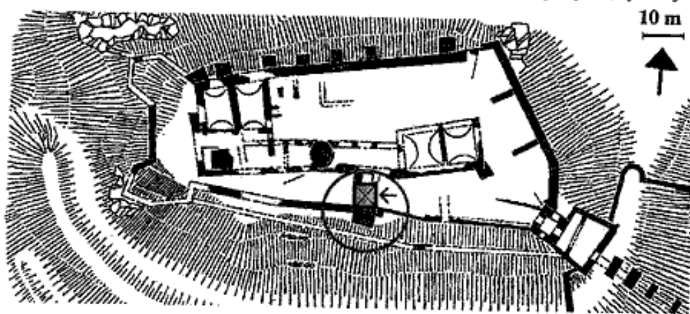
Hrad Lukov, schematický půdorys hradního jádra s vyznačením polohy jižní brány. Šipka označuje vstupní průčelí brány, nalevo od objektu brány se nachází plocha jižního parkánu (podle: Kohoutek 1995, obr. 59).
