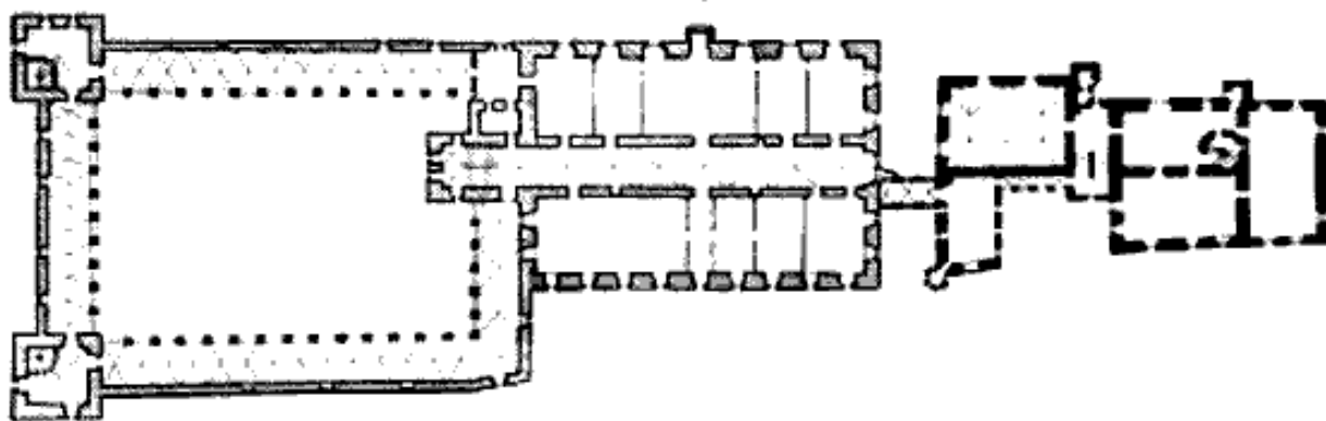
Stockalper, půdorys zámku. Černé zdivo gotické, světlé zdivo renesanční (převzato z monografie Stockalper castle at Brig, 1966).
