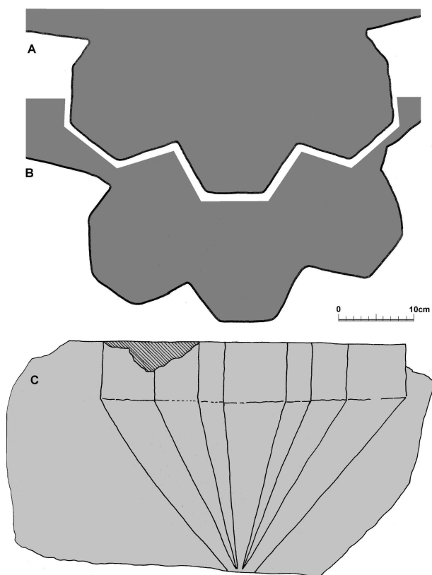
Obr. 5: Hrad Buchlov, zaměření dvojice klenebních konzol z hradního lapidária; A, B – zaměření horní hrany prvků, C – čelní pohled na spodní z nich (Vrla 2015).
