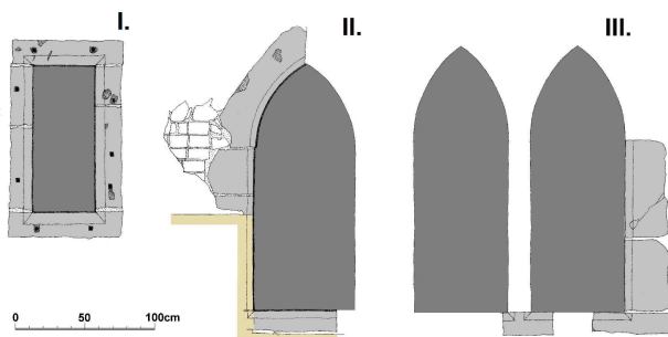
Obr. 4: Hrad Buchlov, zaměření vybraných okenních ostění z 2. poloviny 13. stol.; I – východní věž (zazděné okno v západní zdi), II, III – severní fasáda palácového traktu (Vrla 2015).
