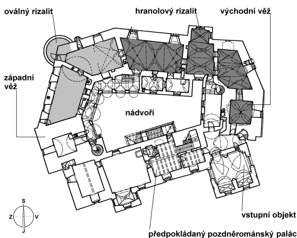
Obr. 2: Hrad Buchlov, půdorys patra hradního jádra s vyznačením částí, zmiňovaných v textu. Šedě jsou vyznačeny prostory zkoumaného severního traktu; tmavý odstín šedé – stávající prostory s dochovanými pozdněgotickými klenbami, světlý odstín šedé – pokus o rekonstrukci dispozice západní části traktu pro období přelomu 15. a 16. stol., včetně náznaku možné podoby části zaniklých kleneb (Vrla 2012).
