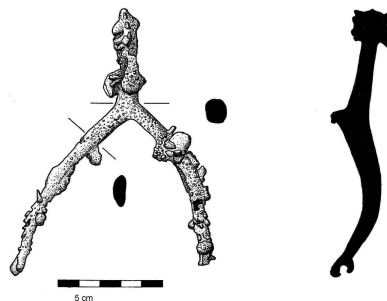
Ostruha z hradu Landštejna (kresba autor 2015).
