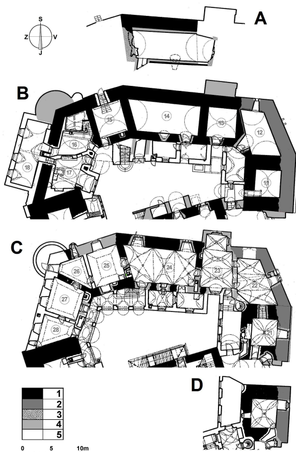
Obr. 3: Hrad Buchlov, půdorysy jednotlivých úrovní severní části jádra hradu se zjednodušenou analýzou stáří zdí; A – sklep, B – přízemí, C – 1. patro, D – 2. patro (východní věž); 1 – zdivo z období od 1. poloviny 13. do počátku 14. stol., 2 – zdivo nedokončené přestavby z 2. poloviny 15. stol., 3 – skála, 4 – zdivo velké pozdně gotické přestavby, konec 15., počátek 16. stol., 5 – pozdější zdivo (Vrla 2015).
