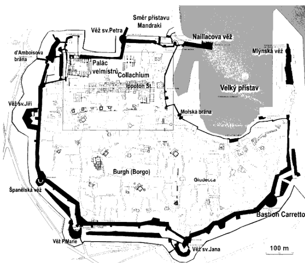
Rhodos, schéma opevnění historické části města (citace v pozn. 8, upraveno).
