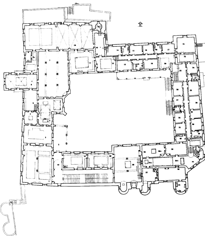
Rhodos, půdorys 1. patra Paláce velmistřů (citace v pozn. 8).
