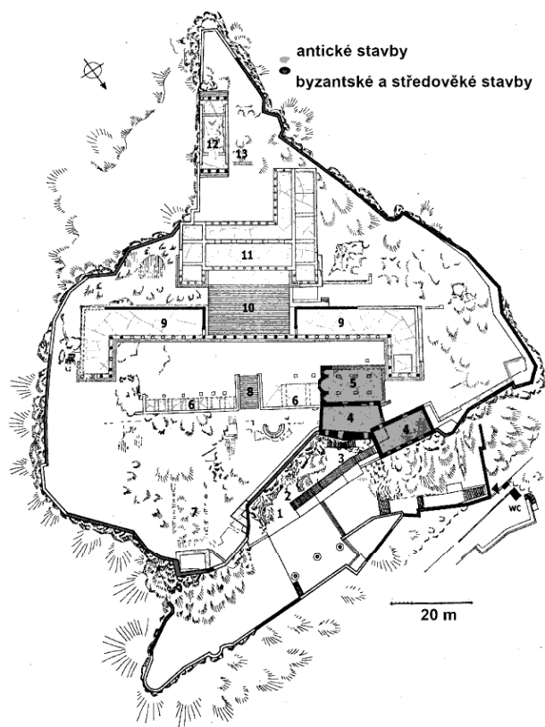
Lindos, půdorys hradiště (reprofoto autor).
