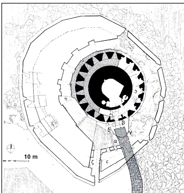
Rhodos, Pevnost sv. Mikuláše, půdorys pevnosti (citace v pozn. 8, s. 71).
