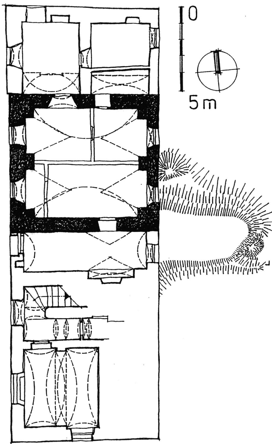
Obr. 23: Veselá - plán přízemí objektu. Renesanční jádro označeno plně.
