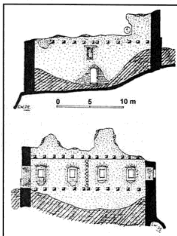
Košťálov. Nahoře: vnitřní líc západní stěny obytné věže. Dole: vnitřní líc východní stěny obytné věže. Stav v r. 1975, měřítko přibližné.
