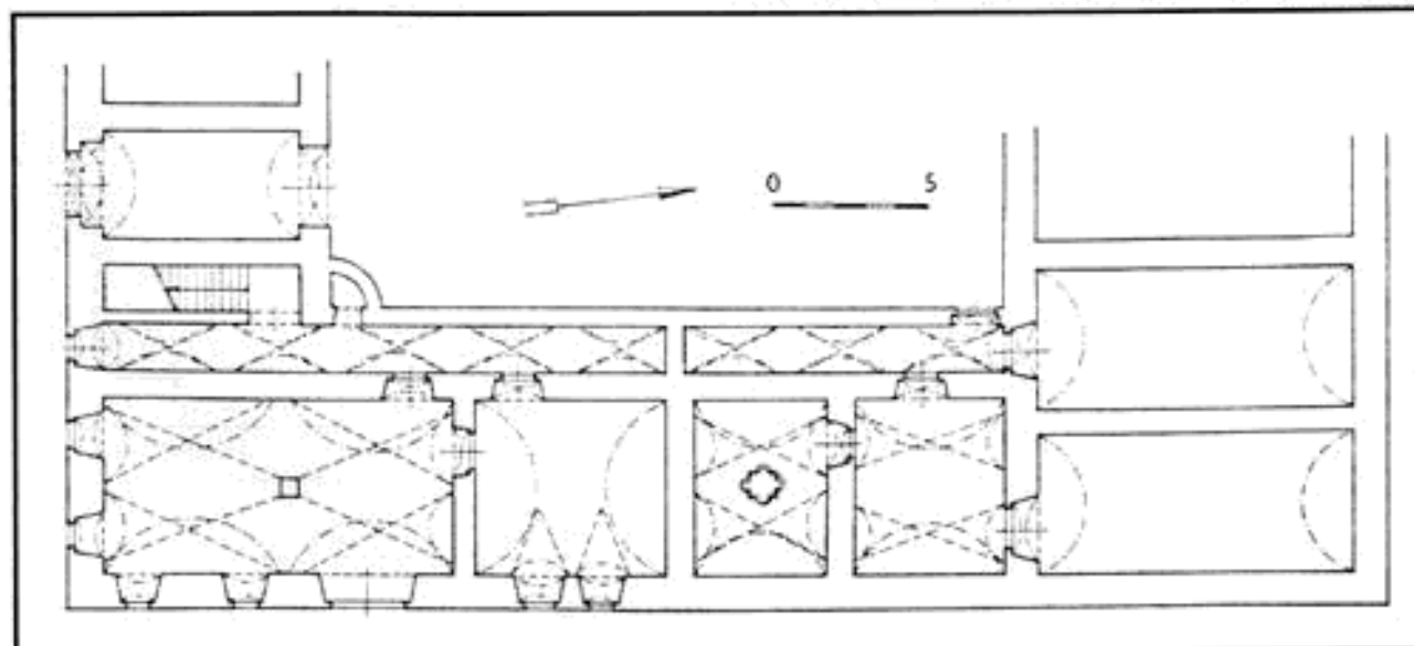
Radiměř - schematický půdorys tvrze podle zaměření Z. Fišery. Kresba J. Sadílek
