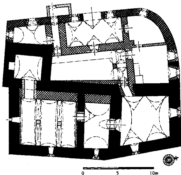
Analytický plán přízemí/suterénu tvrze Měcholupy. Černě zdivo gotické, hustě křížem šrafované pozdně gotické, řídké křížem šrafované renesanční, ostatní mladší (kresba P. Chotěbor – převzato z Encyklopedie českých tvrzí II, 2000, s. 456).
