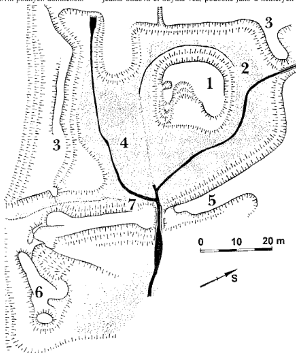
Tvrziště Škodějov. 1 - plošina vlastního tvrziště, 2 - příkop kolem tvrze, 3 - zbytky venkovních valů, 4 - rybník, 5 - násep rybníka, 6 - blíže neurčený terénní relikt, 7 - místo nálezu středověké šipky. Zaměření autor 1995.
