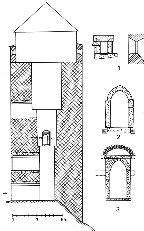
Obr. 2 – Hasištejn (okr. Chomutov). Řez bergfritem (označení stáří zdiv viz obr. 1) a detaily: 1 – nákras ostění renesanční střílny při pohledu z interiéru věže a řez střílnou, 2 – vstupní portálek do věže při pohledu z exteriéru, 3 – vstupní portálek do věže při pohledu z interiéru. Rozlišení stáří zdiv viz popiska obr. 1.
