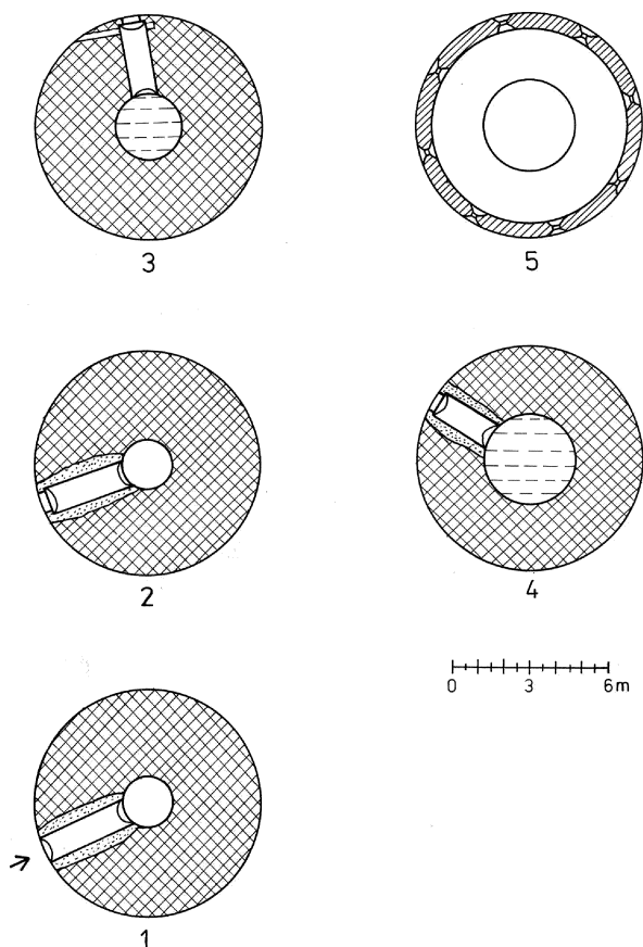
Obr. 1: Hasištejn (okr. Chomutov). Půdorysy jednotlivých podlaží bergfritu. Křížkovaně zdivo z počátku 14. století, šrafovaně zdivo z přelomu 15. a 16. století, tečkovaně zdivo z let 1891 – 1892.
