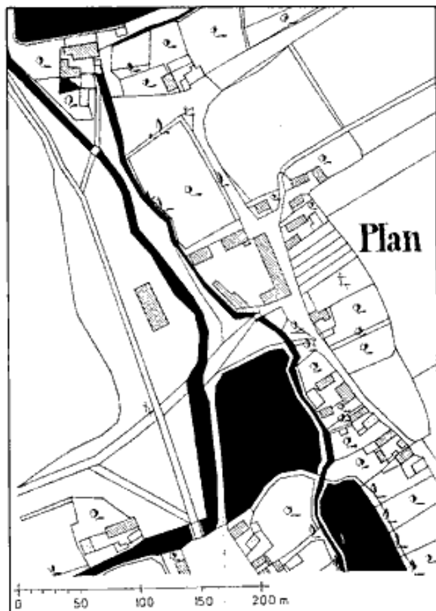
Stoppelhof (okr. Most), výřřez z katastrální mapy vsi z r. 1842. Poplužní dvůr je rozložen při levém břehu mlýnského náhonu, přibližně uprostřed vesnické zástavby. její jižní okraj náležřř již ke Kopistům. Šřřafami značeny budovy z nespáleného a tečkami budovy ze spáleného materiálu, plně vodní plochy a toky (kresba autor)
