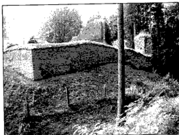
Opravené zdivo severovýchodního nároží a severní zdi bastionu, vnější líc, po dokončení prací (září 2008)
