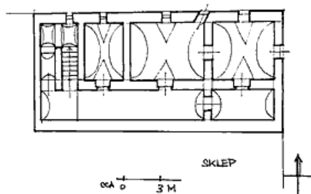
Hochperk (Křiše čp. 59) – neměřené schéma půdorysu (T. Karel 2002)
