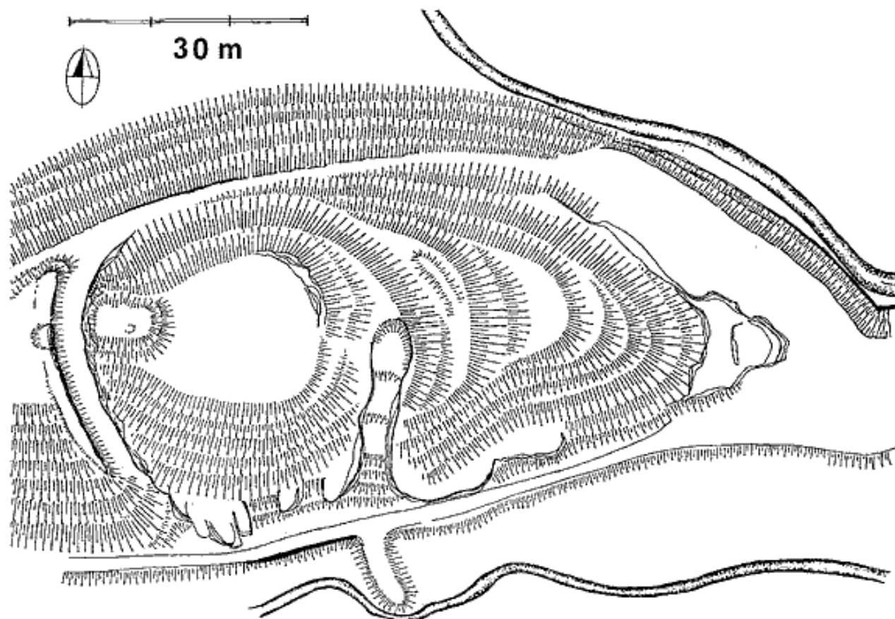
Hrad Milkov, náčrt situace, březen 2007 (zaměření a kresba autor)
