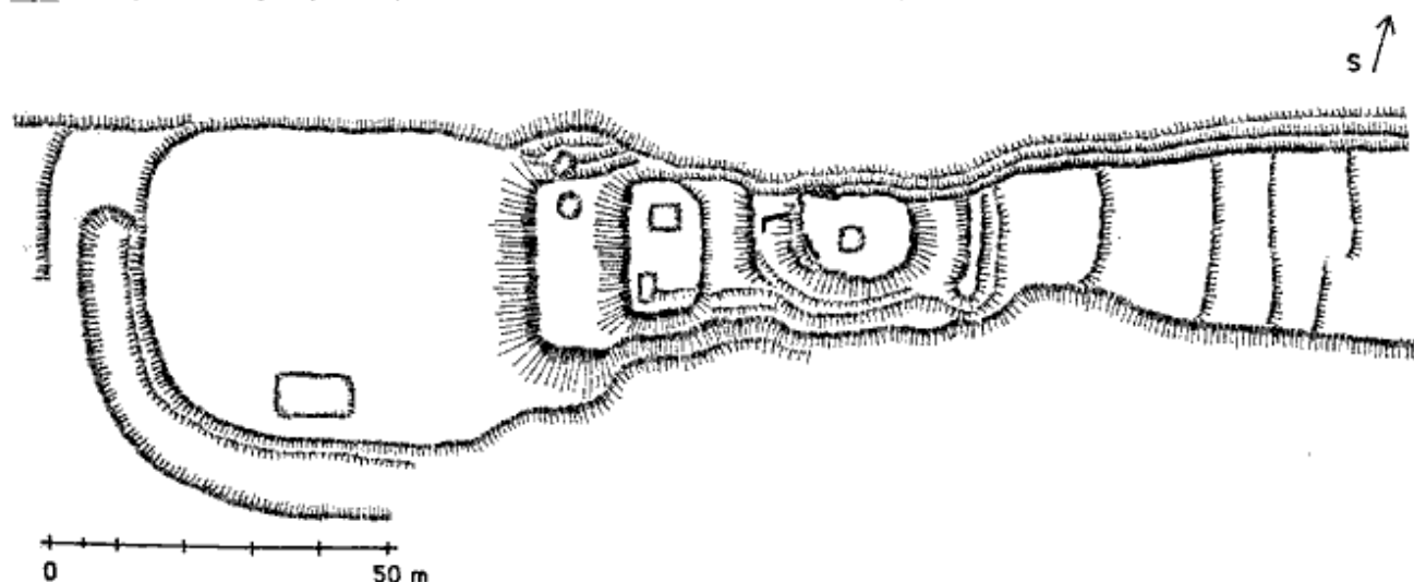
Paradies (o. Teplice), celkový plán hradu bez parkánu pod severním svahem, který nebyl pro značný výškový rozdíl měřen. Stav 12. prosince 2002, zaměření a kresba autor
