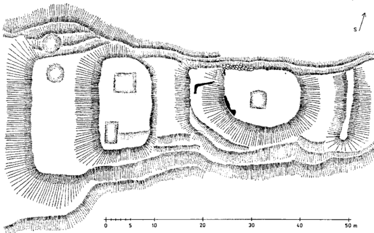
Paradies (o. Teplice), plán jádra hradu s menším západním předhradím. Stav 12. prosince 2002, zaměření a kresba autor
