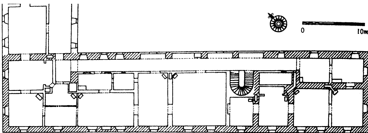
Přízemí jižního (jihozápadního) křídla zámku na plánu z doby kolem r. 1900. Šrafované předpokládané renesanční zdivo (kresba J. Úlovec, Kolektiv: Encyklopedie českých tvrzí II. Praha 2000, s. 306).
