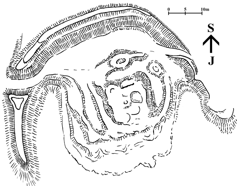
Obr. 2: Plán tvrže. Za zaměření pásmem děkujeme sl. Martině Kosířové, studentce II. ročníku Geodézie a kat. nem. na SPŠ stavební v Českých Budějovicích (kresba Jakub Vazač 2017).
