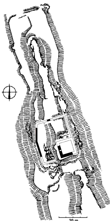
Obr. 1: Netřeb (okr. Domažlice) – půdorysný plán hradu dle Z. Procházky (Durdík, T. – Sušický, V.: Zříceniny hradů, tvrzí a zámků. Západní Čechy. Praha 2005, s. 123–124. Úprava autor).
