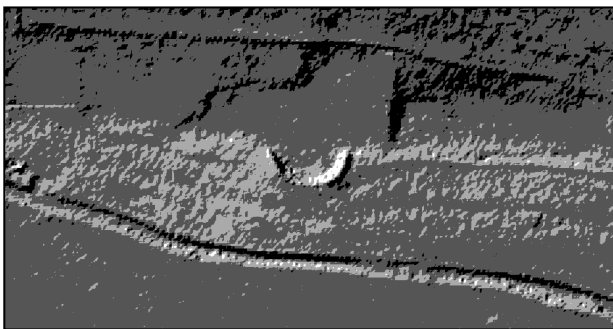
Obr. 4: Tvrziště Očín – stínovaný reliéf podle serveru Analýzy výškopisu ( https://ags.cuzk.cz/dmr/ ).
