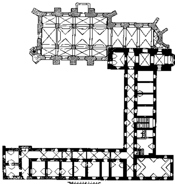
Klášter sv. Dobrotivá, půdorys (citace v pozn. 15, s. 6).
